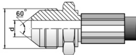
JIS-(Ш) ниппель с наружной резьбой
